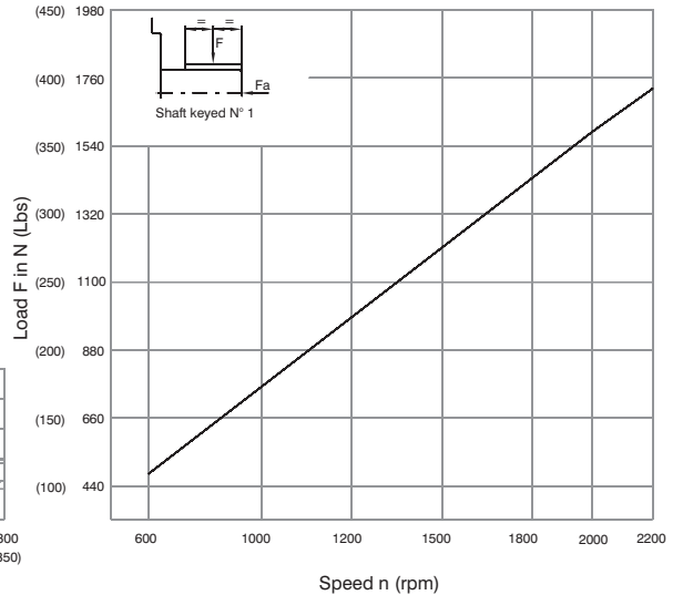
PERMISSIBLE RADIAL LOAD
