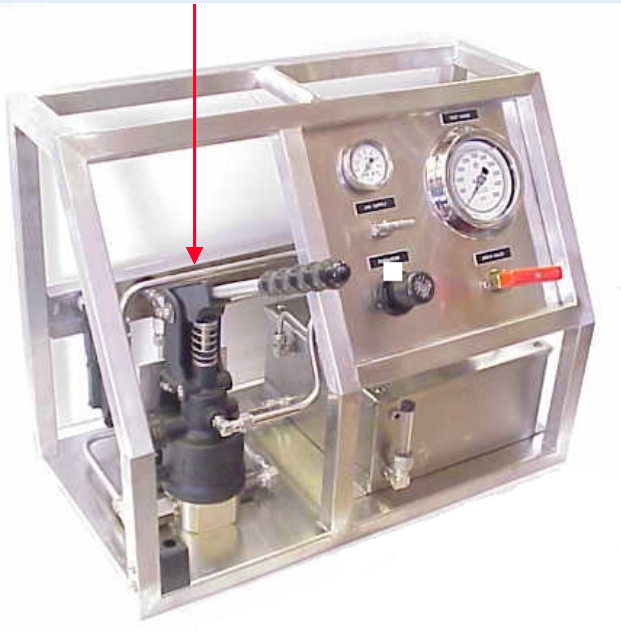
Minipump
